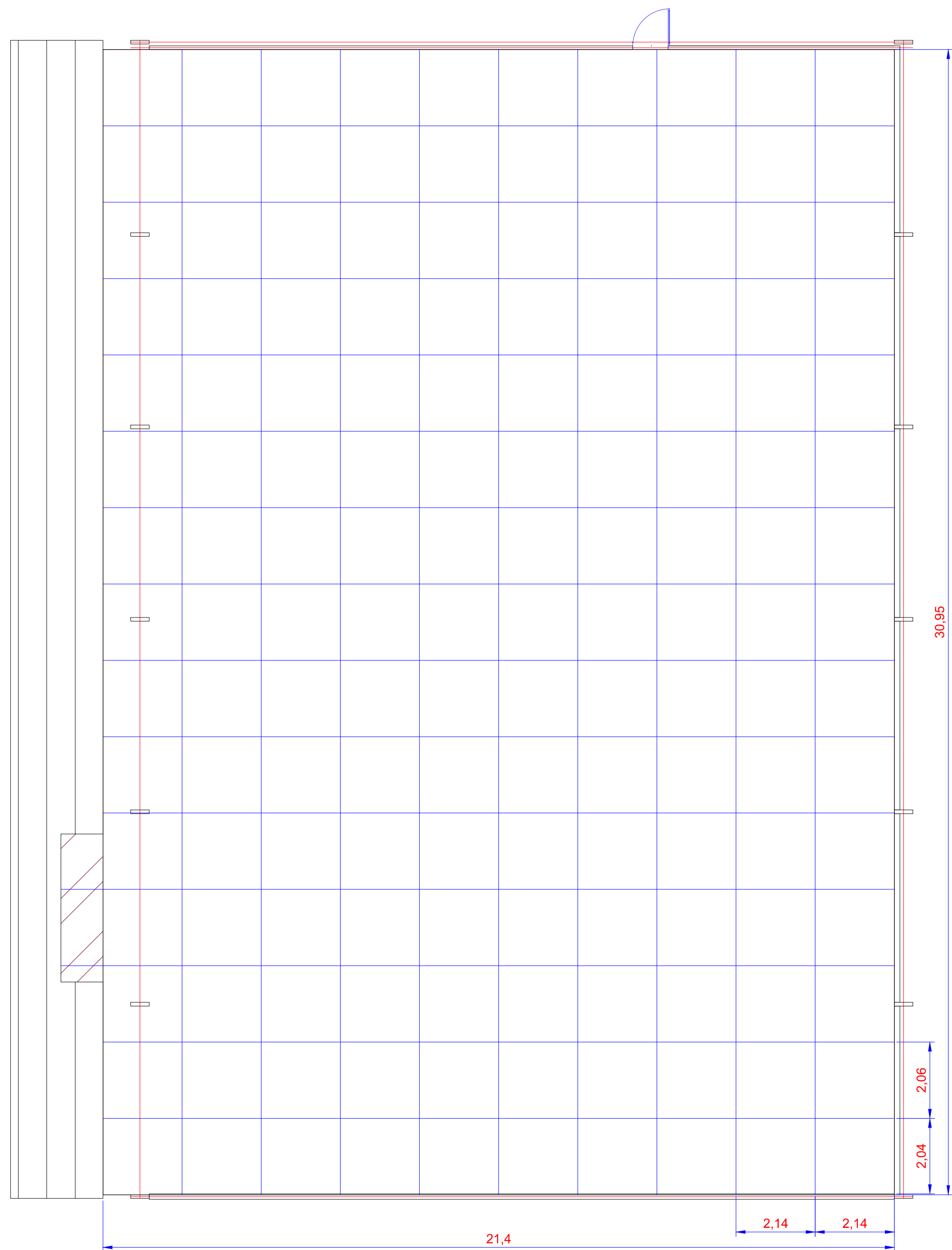
VISTA EM PLANTA ESCALA 1:100
