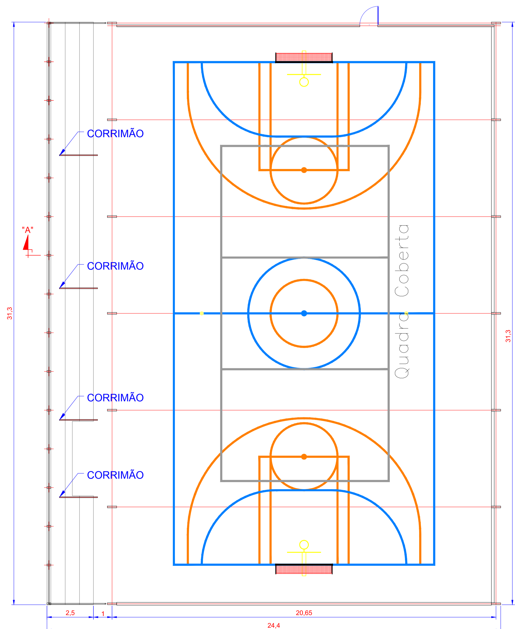
VISTA EM PLANTA ESCALA 1:100
