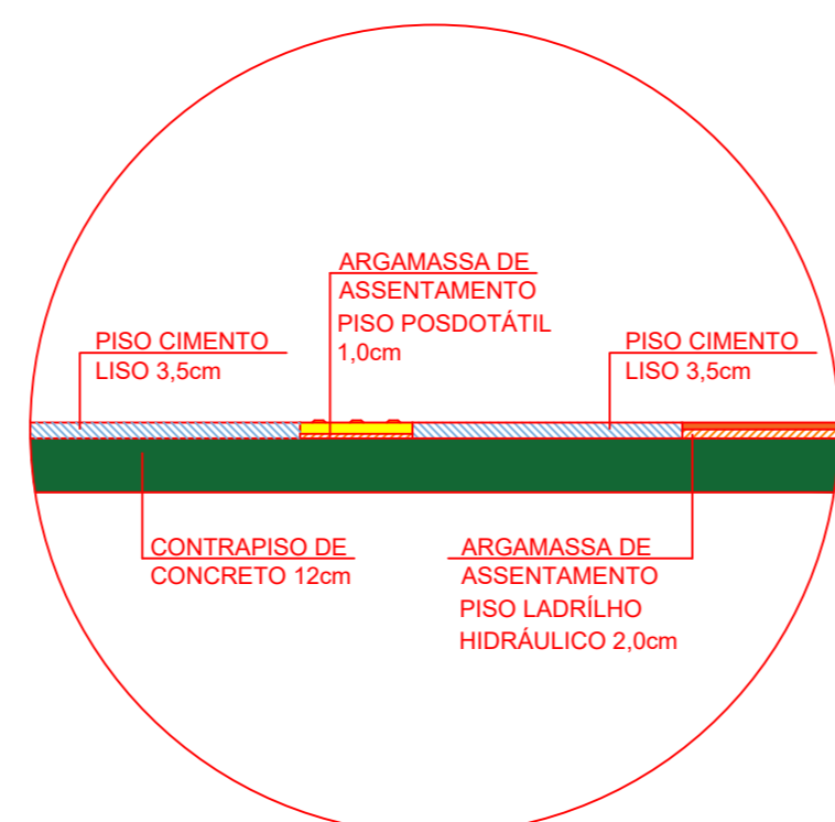
DETALHE ESPESSURAS CALÇADA SEM ESCALA
