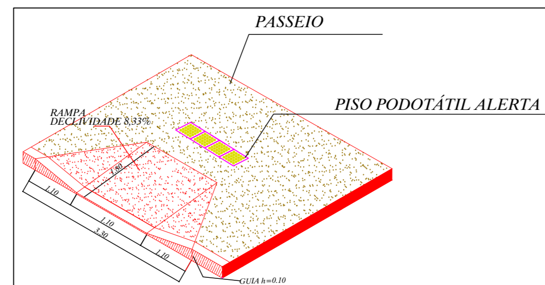
RAMPA PARA PORTADORES DE NECESSIDADES ESPECIAIS
