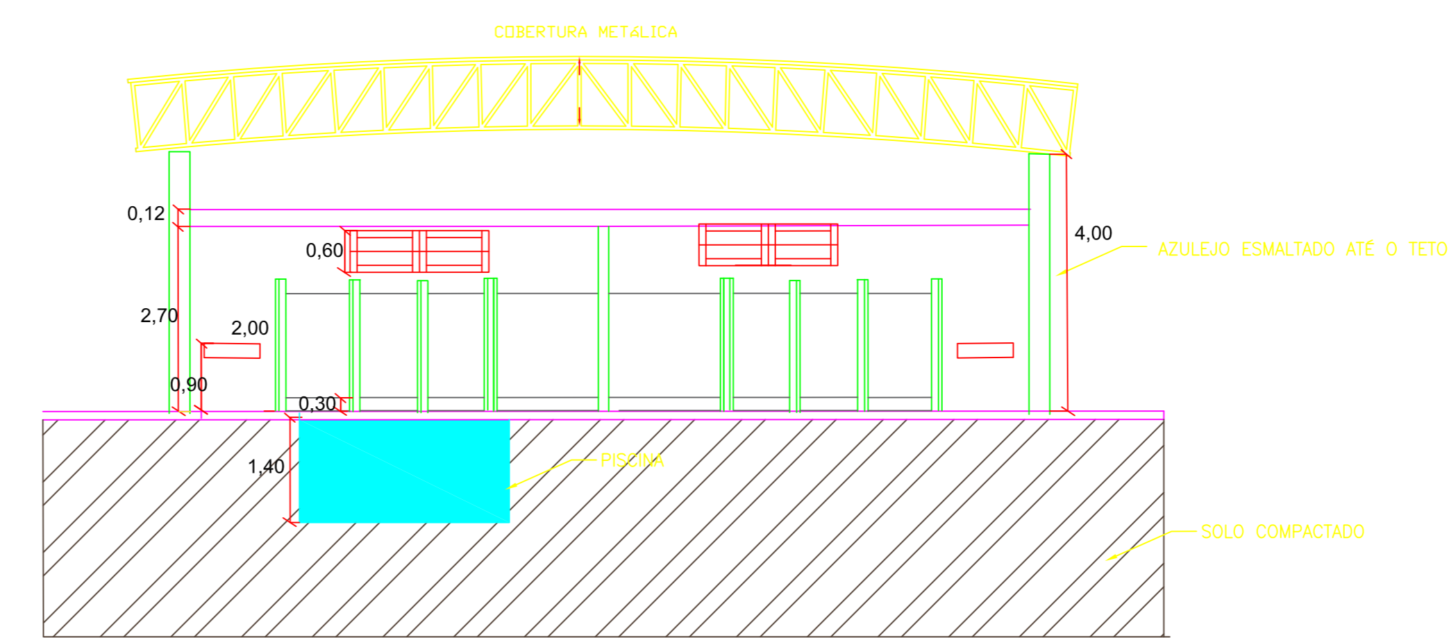
CORTE ESQUEMÁTICO - AA (VESTIÁRIO) SEM ESCALA
