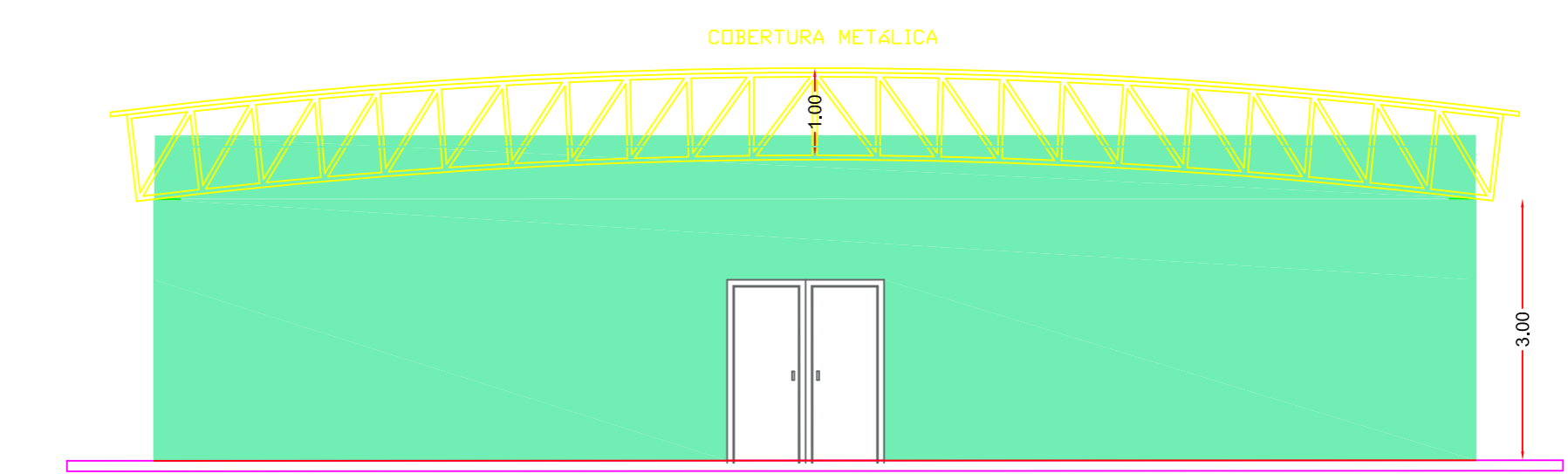
FACHADA ESCALA 1:100
