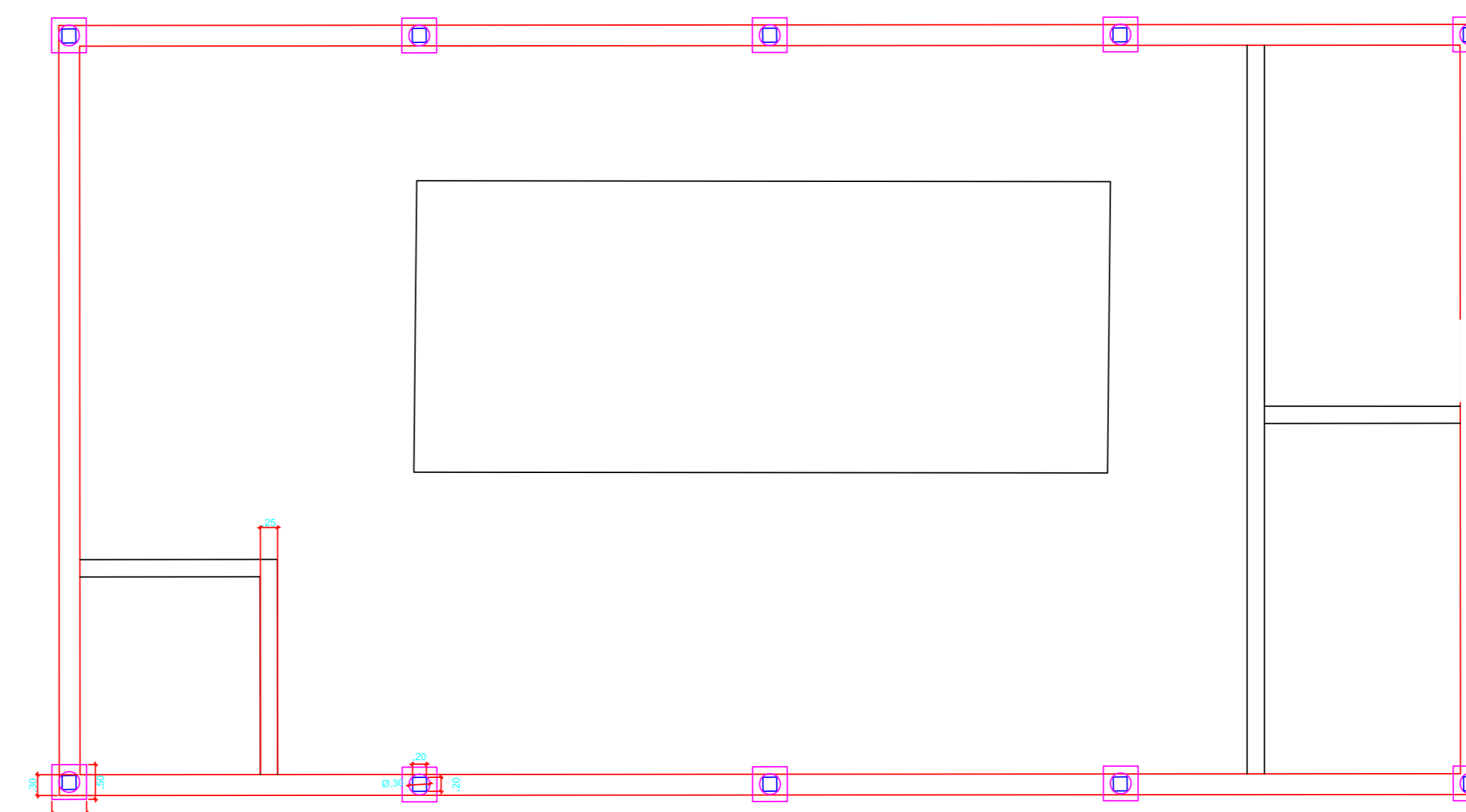
FUNDAÇÃO – BLOCOS, ESTACAS E BALDRAMES ESCALA 1:100
