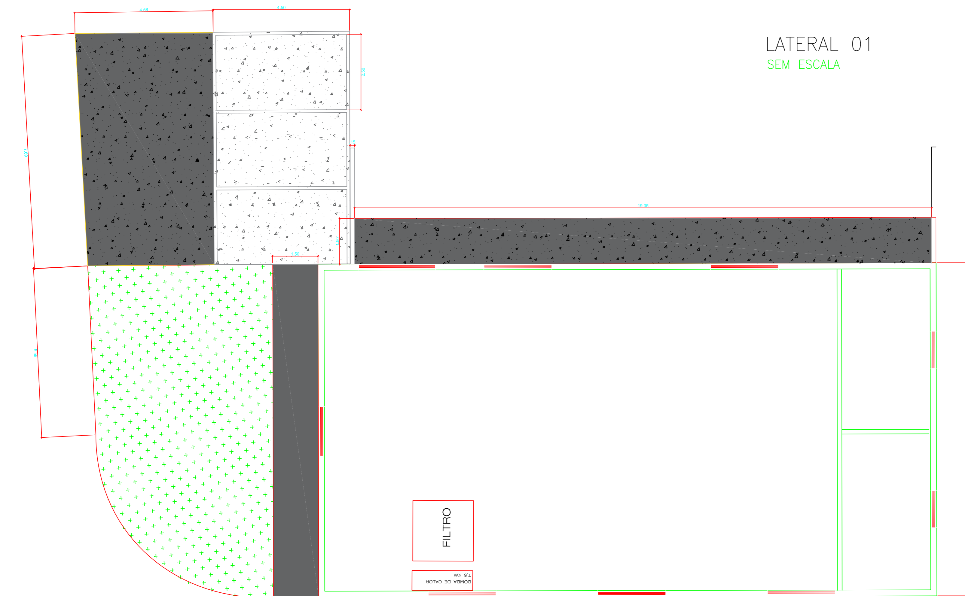
PLANTA BAIXA - ÁREA EXTERNA ESCALA 1:100
